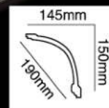
HG-7675-1 規格 (Spec): 145X150 mm
