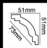
HG-7503 长度(Long):2400mm 面宽(Breath):73mm
