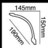
HG-7676 長度 ( Long ) :2400 mm 面寬 ( Breath ) :190 mm 對花 ( Pattern ) :1140 mm
