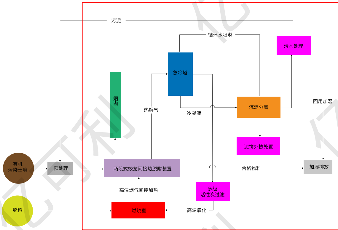
螺旋热脱附工艺流程图
